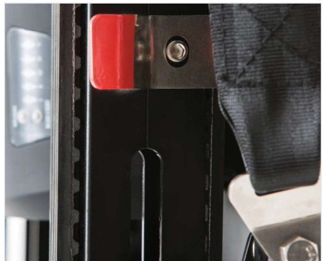
■ System zum Lösen der Raupenverankerung
